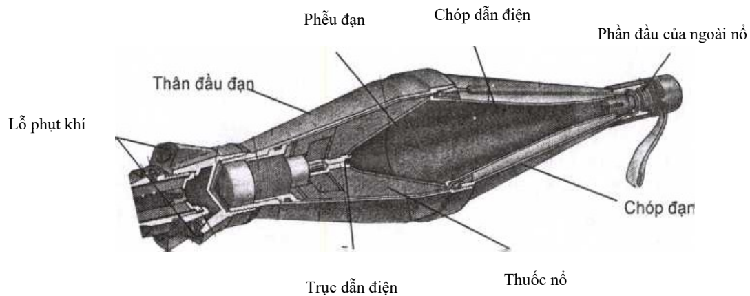
Hình 12.54. Đầu đạn
