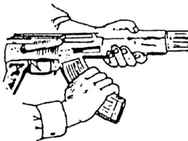
Hình 12.65. Tháo hộp tiếp đạn, kiểm tra súng
