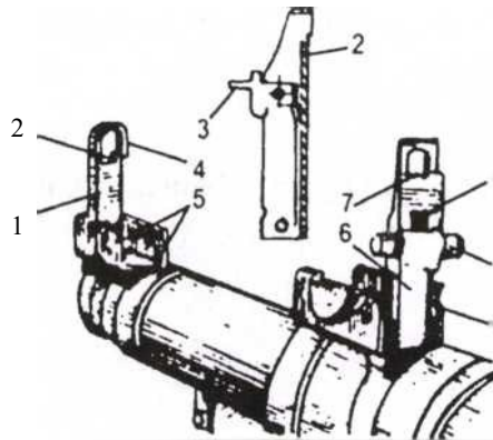
Hình 12.48. Bộ phận ngắm cơ khí
