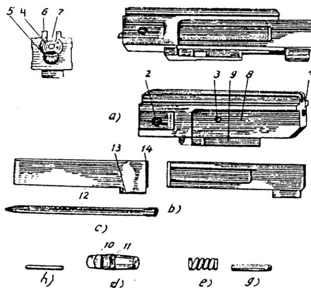
Hình 12.40. Khóa nòng
