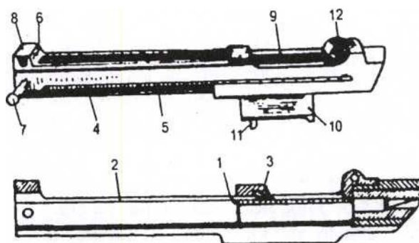
Hình 12.37. Hộp khoá nòng
