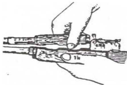
Hình 12.71. Tháo ống dẫn thoi và ốp lót tay trên
