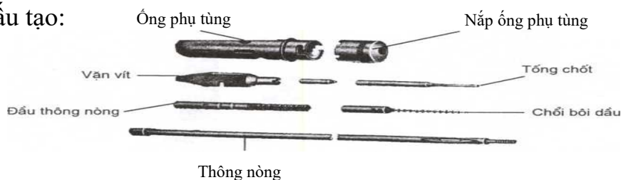
Hình 12.31. Phụ tùng
