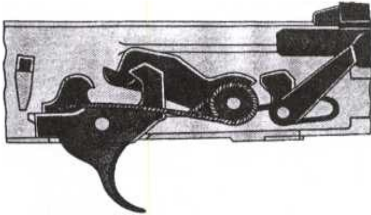
Hình 12.33. Vị trí các chi tiết bộ phận cò khi bắn phát một
