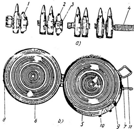
Hình 12.44. Băng đạn và hộp băng
