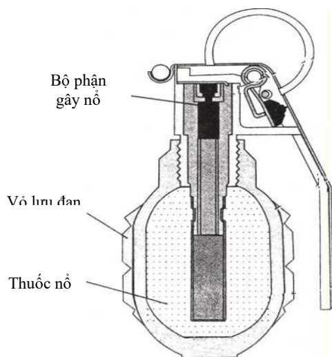
Hình 12.58. Lựu đạn cần 97
