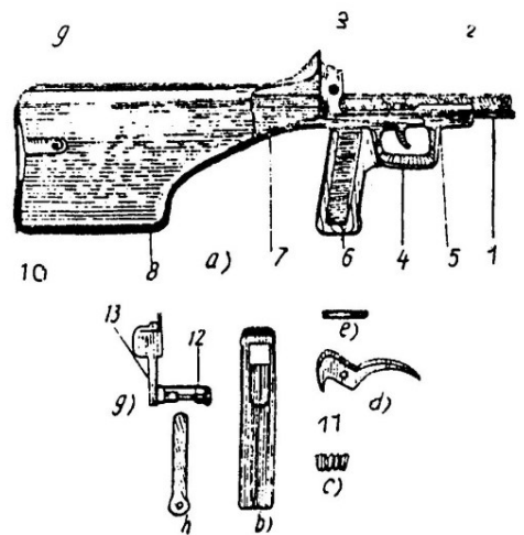
Hình 12.42. Bộ phận cò và báng súng
