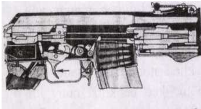
Hình 12.32. Vị trí các chi tiết bộ phận cò khi bắn liên thanh
