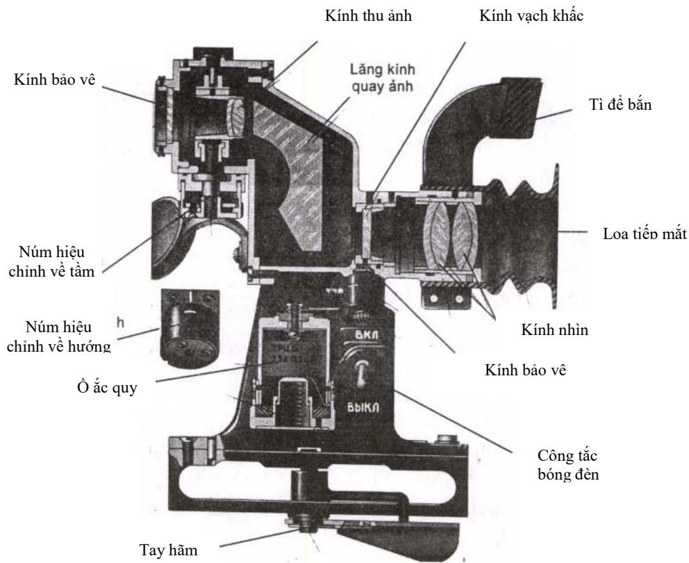
Hình 12.51. Kính ngắm quang học
