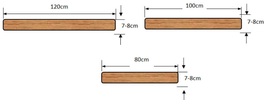
Hình 13.16. Bộ nẹp đùi bằng gỗ
