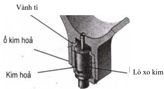
Hình 12.50. Kim hoả
