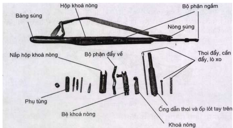
Hình 12.2: Cấu tạo của súng trường CKC
