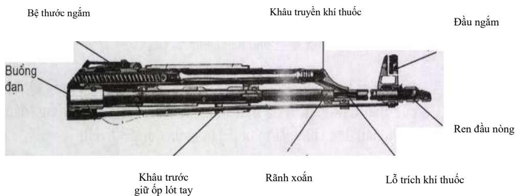
Hình 12.19. Bộ phận nòng súng
