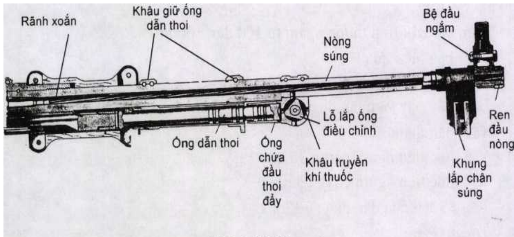
Hình 12.35. Nòng súng
