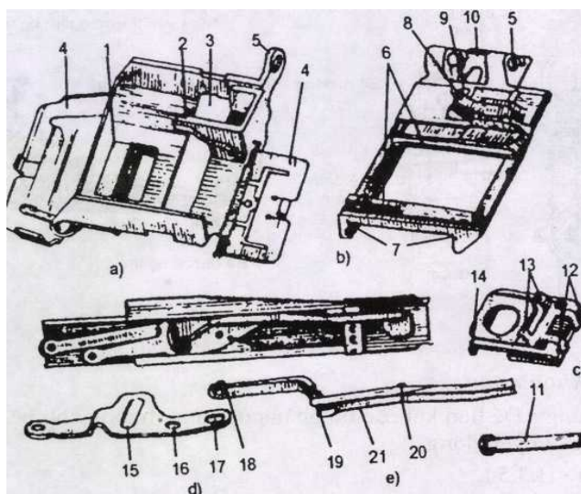
Hình 12.38. Bộ phận tiếp đạn và nắp hộp khóa nòng
