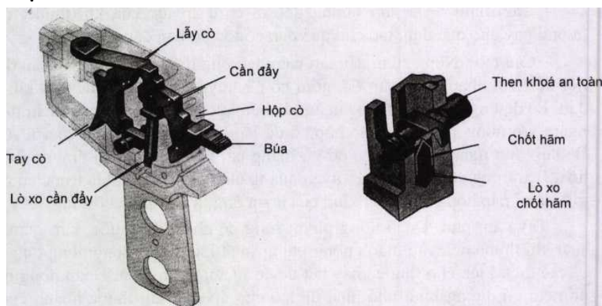
Hình 12.49. Bộ phận cò
