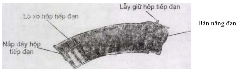
Hình 12.29. Hộp tiếp đạn
