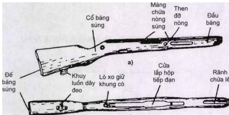
Hình 12.13. Báng súng
