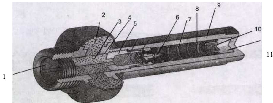
Hình 12.55. Ống thuốc đẩy phản lực
