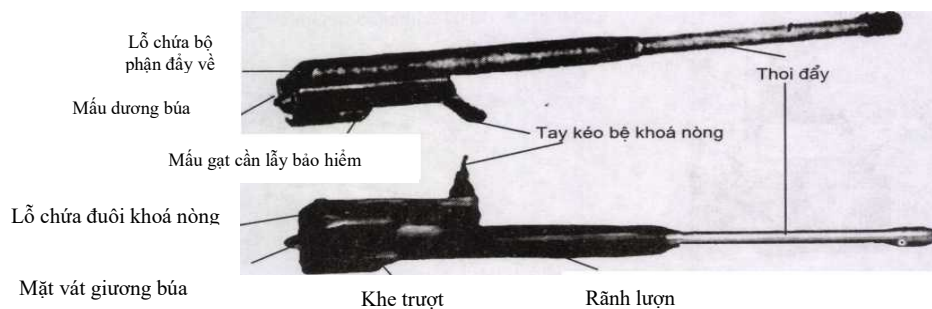
Hình 12.23. Bộ khoá nòng
