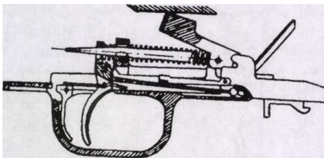
Hình 12.17. Chuyển động các bộ phận khi bắn
