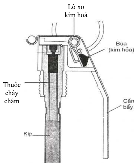
Hình 12.59. Bộ phận gây nổ lựu đạn cần 97
