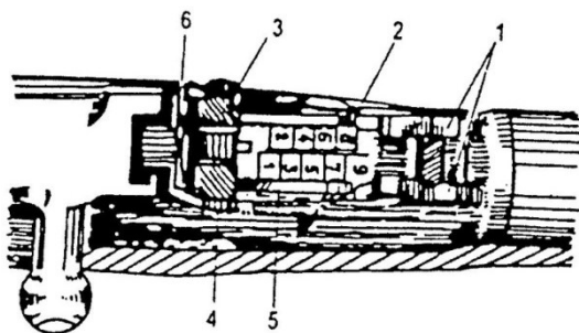
Hình 12.4. Bộ phận thước ngắm
