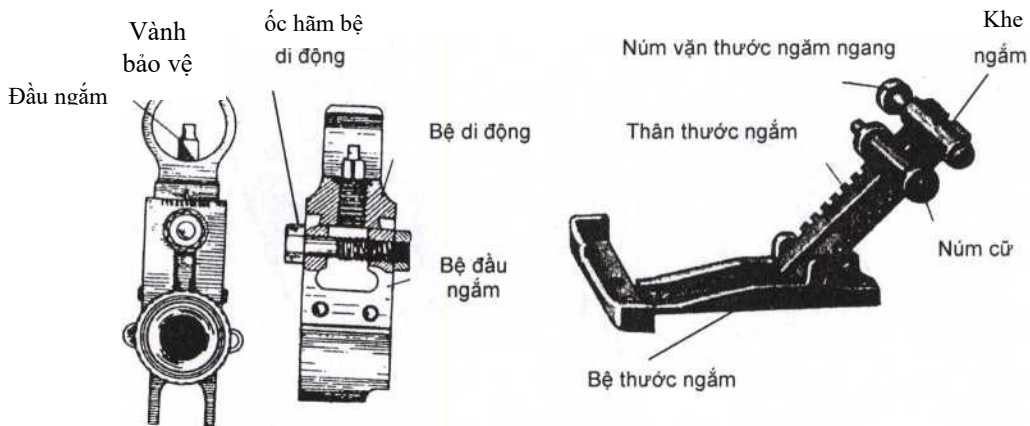
Hình 12.36. Bộ phận ngắm
