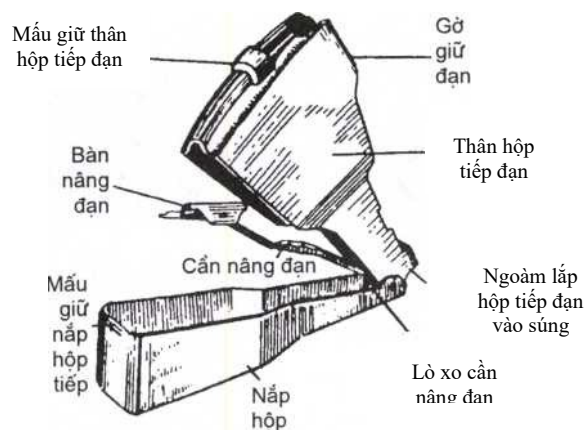
Hình 12.14. Hộp tiếp đạn
