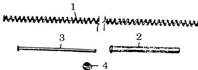
Hình 12.10. Bộ phận đẩy về
