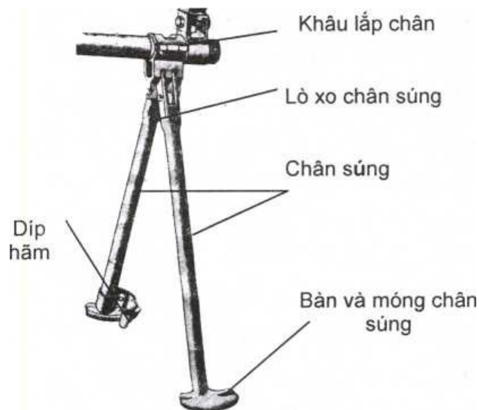
Hình 12.45. Chân súng
