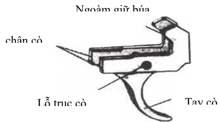
Hình 12.25. Bộ phận cò
