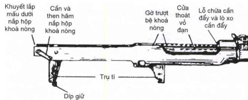
Hình 12.5. Hộp khoá nòng
