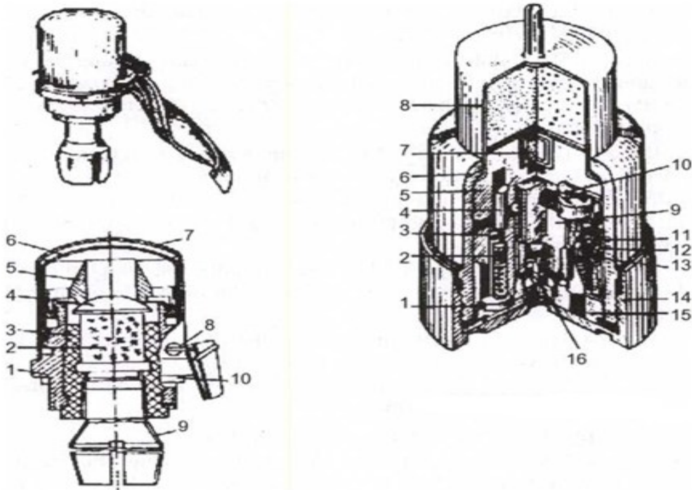
Hình 12.57. Bộ phận sinh điện
