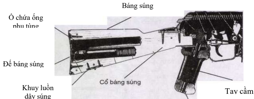
Hình 12.28. Báng súng
