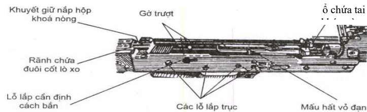
Hình 12.21. Hộp khoá nòng
