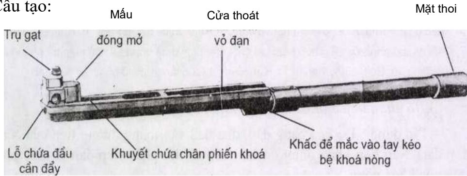
Hình 12.39. Bộ khoá nòng và thoi đẩy
