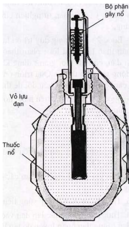
Hình 12.60. Lựu đạn \Phi -1 (phi -1)
