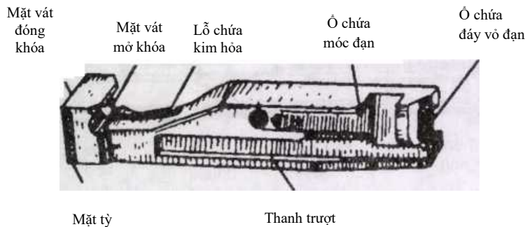
Hình 12.8. Khoá nòng
