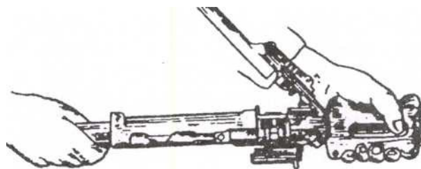
Hình 12.77. Tháo bộ khoá nòng và khoá nòng
