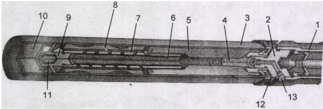
Hình 12.56. Đuôi đạn
