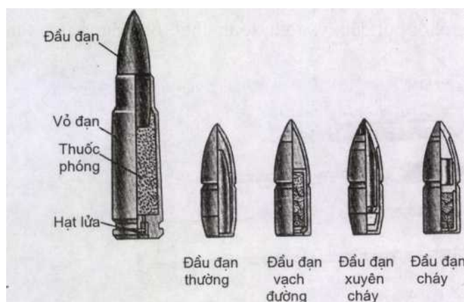
Hình 12.16. Đạn súng tiểu liên (K56)
