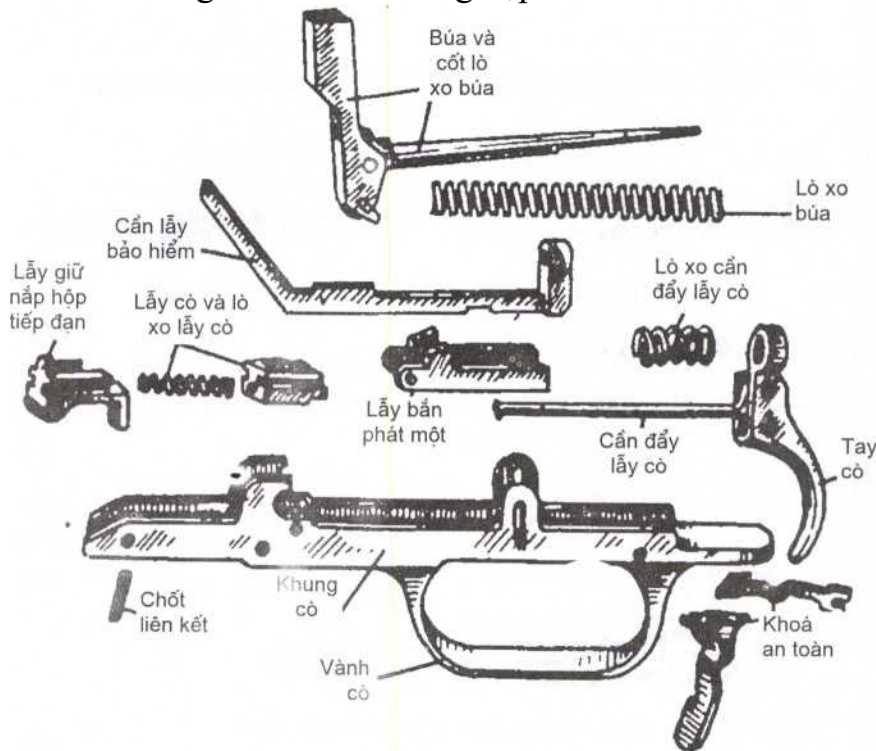
Hình 12.9. Bộ phận cò
