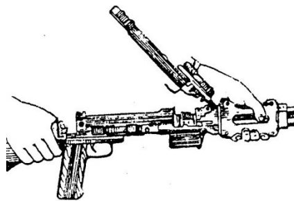
Hình 12.76. Tháo bộ phận cò và báng súng
