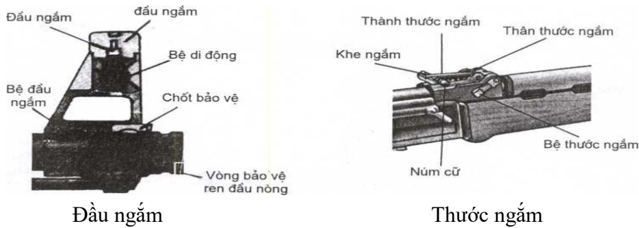
Hình 12.20. Bộ phận ngắm
